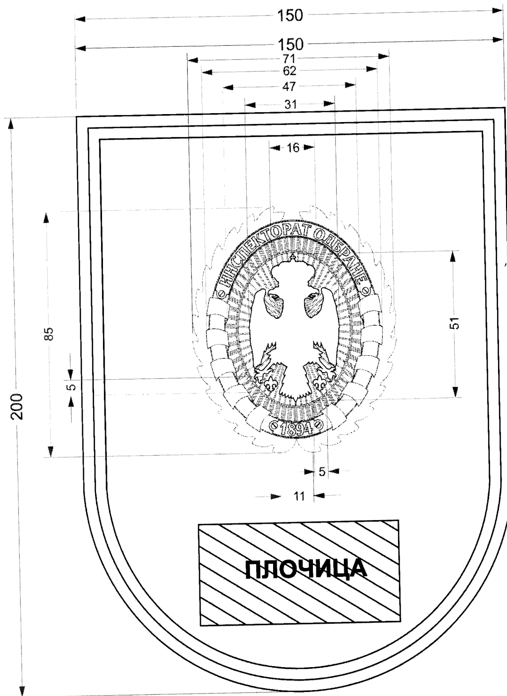
Слика 18. Димензије Плакете Инспектората одбране
